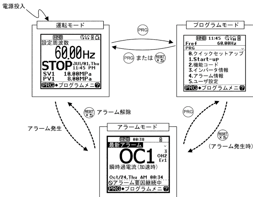
図 2 操作モード状態遷移
