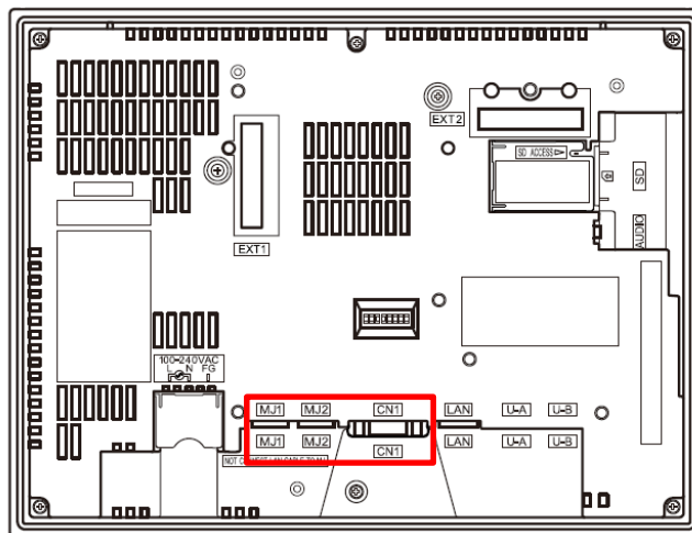
MJ1/MJ2/CN1
